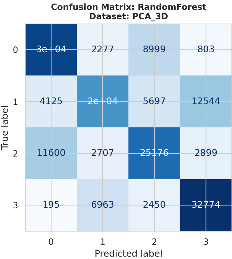
ConfusionMatrix_RandomForest_PCA_3D.png
