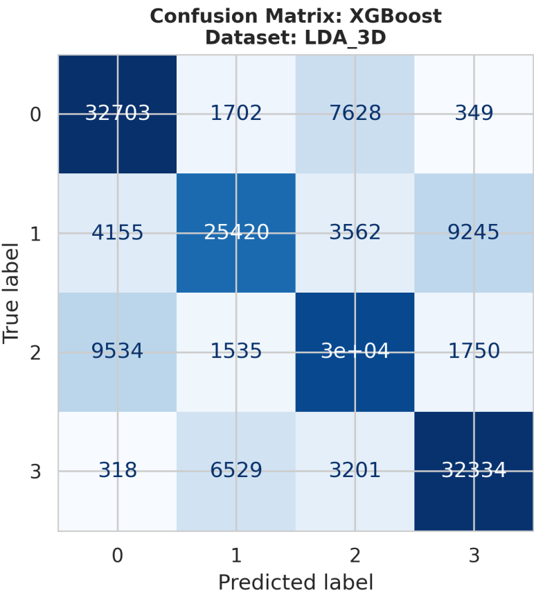
ConfusionMatrix_XGBoost_LDA_3D.png
