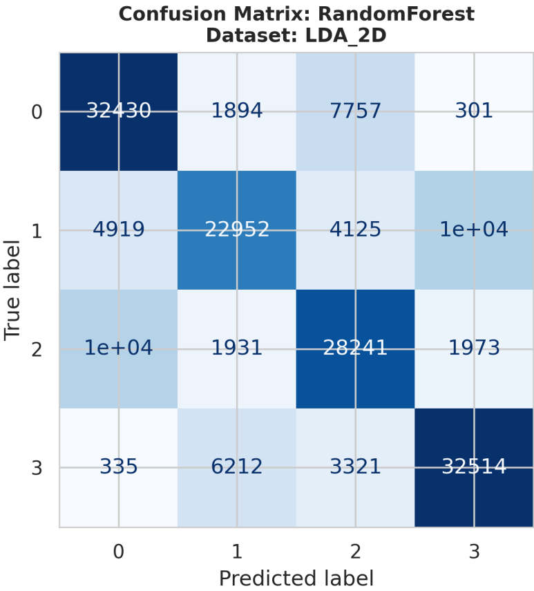
ConfusionMatrix_RandomForest_LDA_2D.png
