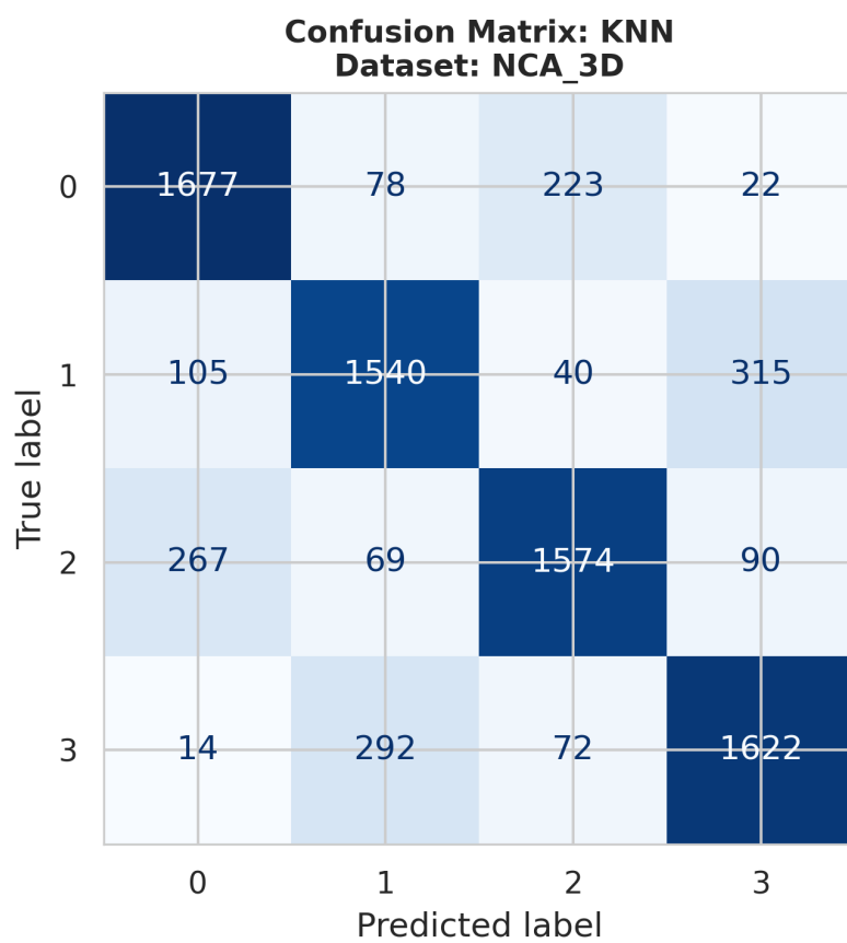
ConfusionMatrix_KNN_NCA_3D.png
