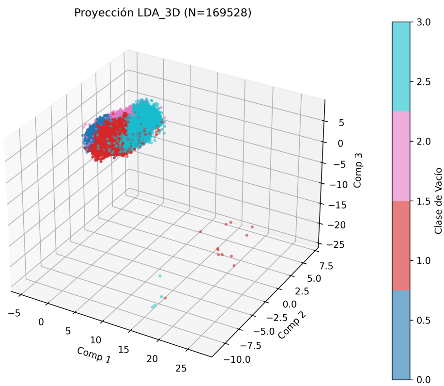
plot_LDA_3D.png
