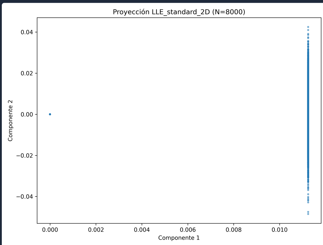
plot_LLE_standard_2D.png
