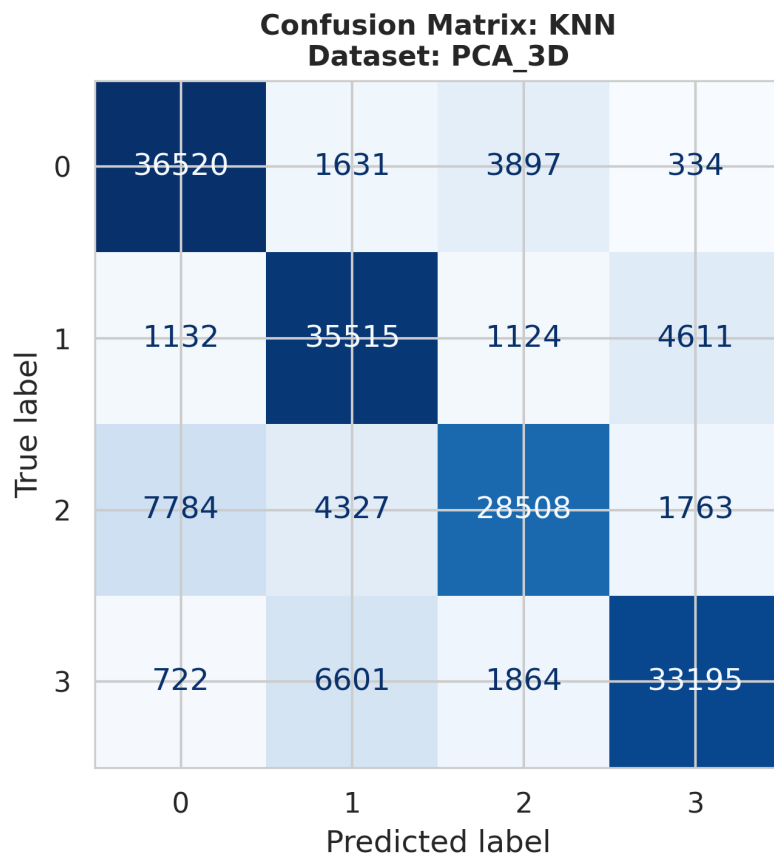
ConfusionMatrix_KNN_PCA_3D.png
