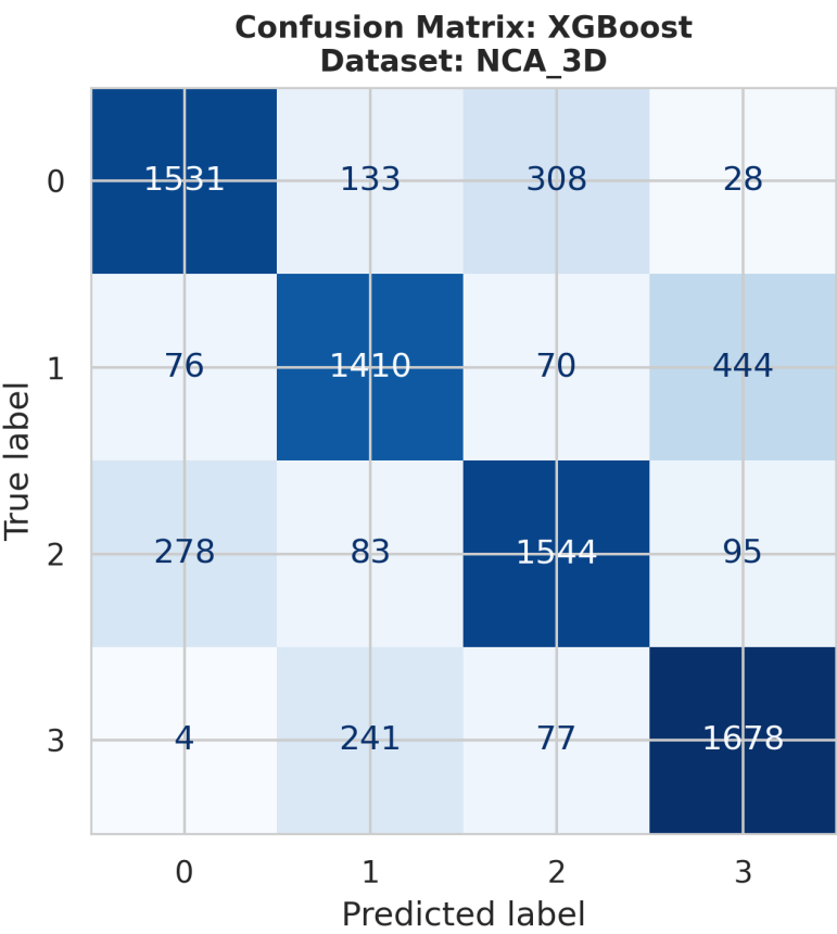
ConfusionMatrix_XGBoost_NCA_3D.png
