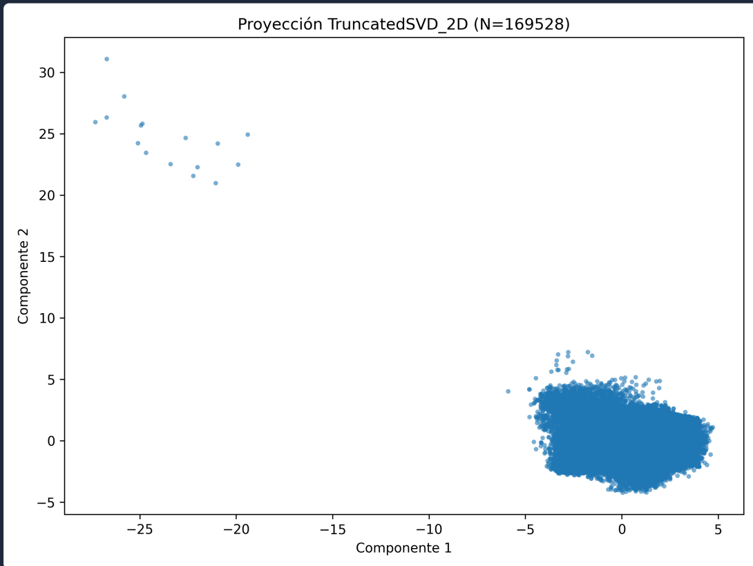
plot_TruncatedSVD_2D.png
