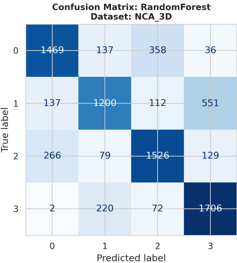
ConfusionMatrix_RandomForest_NCA_3D.png
