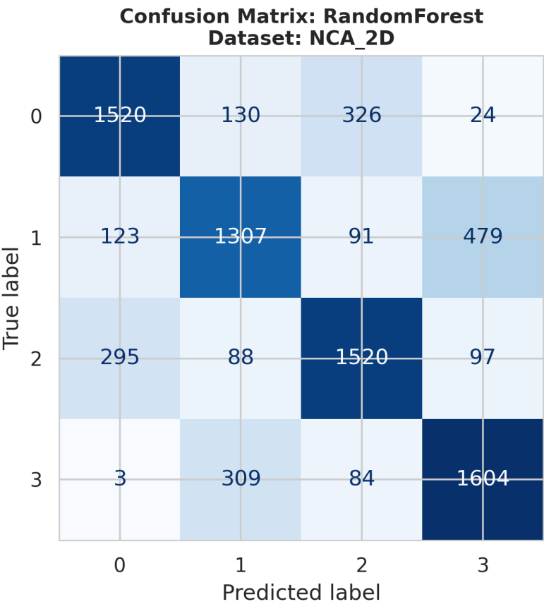
ConfusionMatrix_RandomForest_NCA_2D.png
