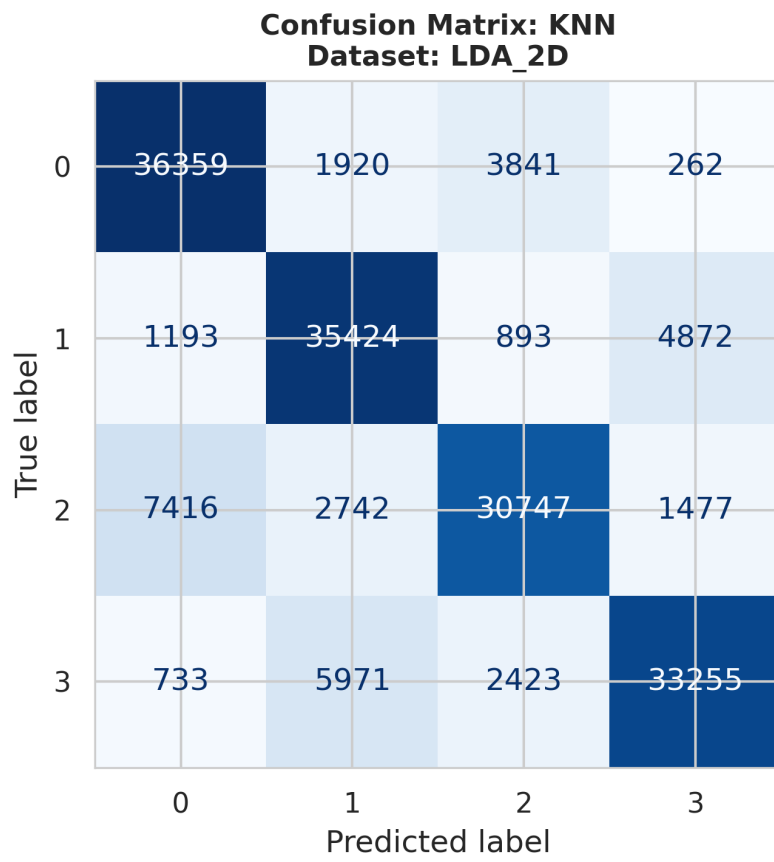
ConfusionMatrix_KNN_LDA_2D.png
