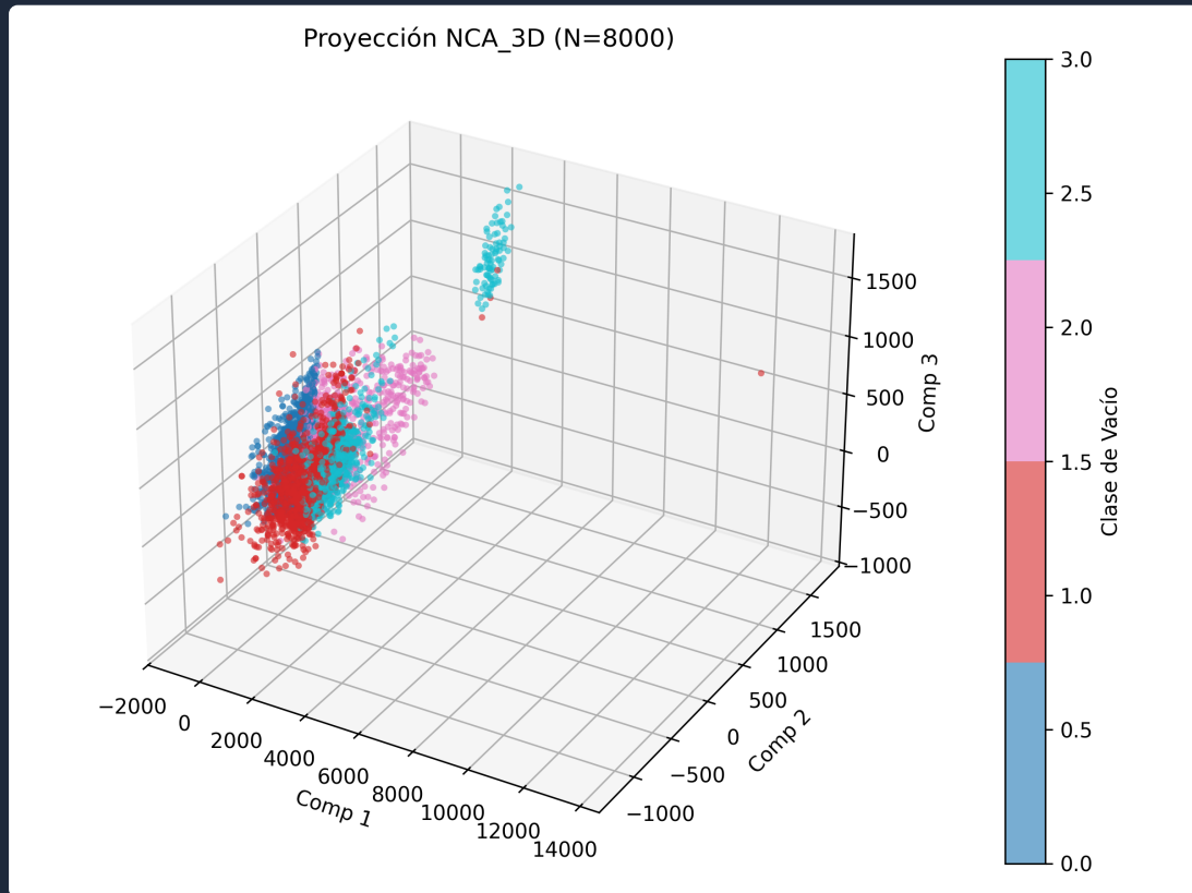
plot_NCA_3D.png
