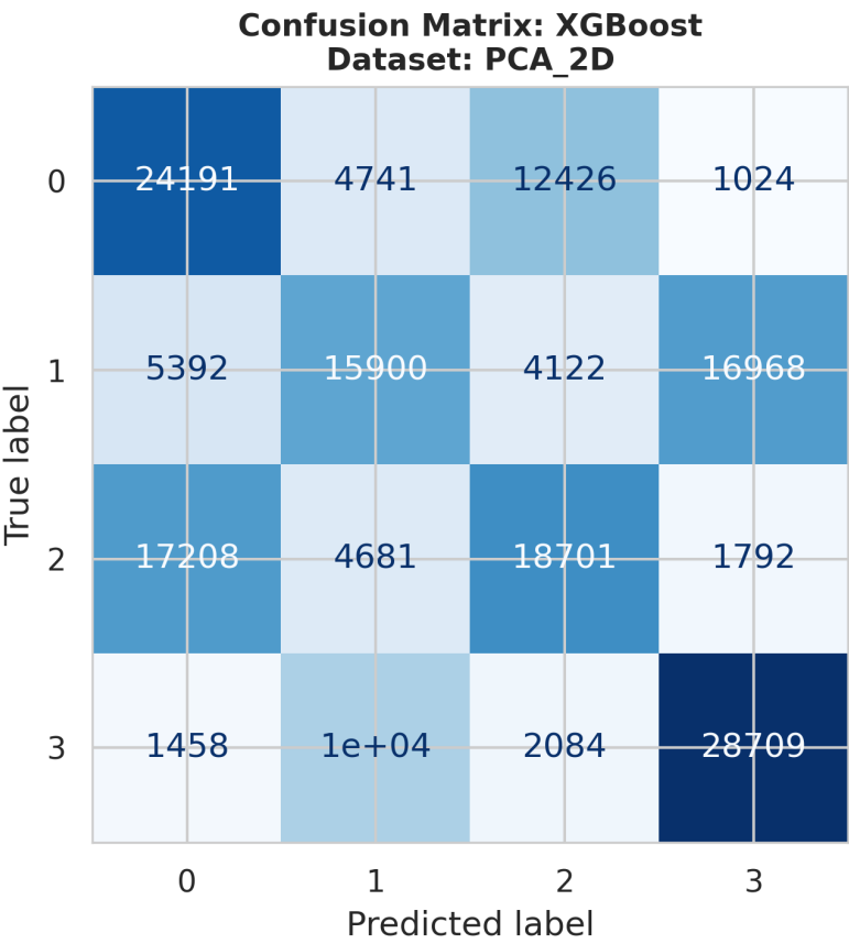
ConfusionMatrix_XGBoost_PCA_2D.png
