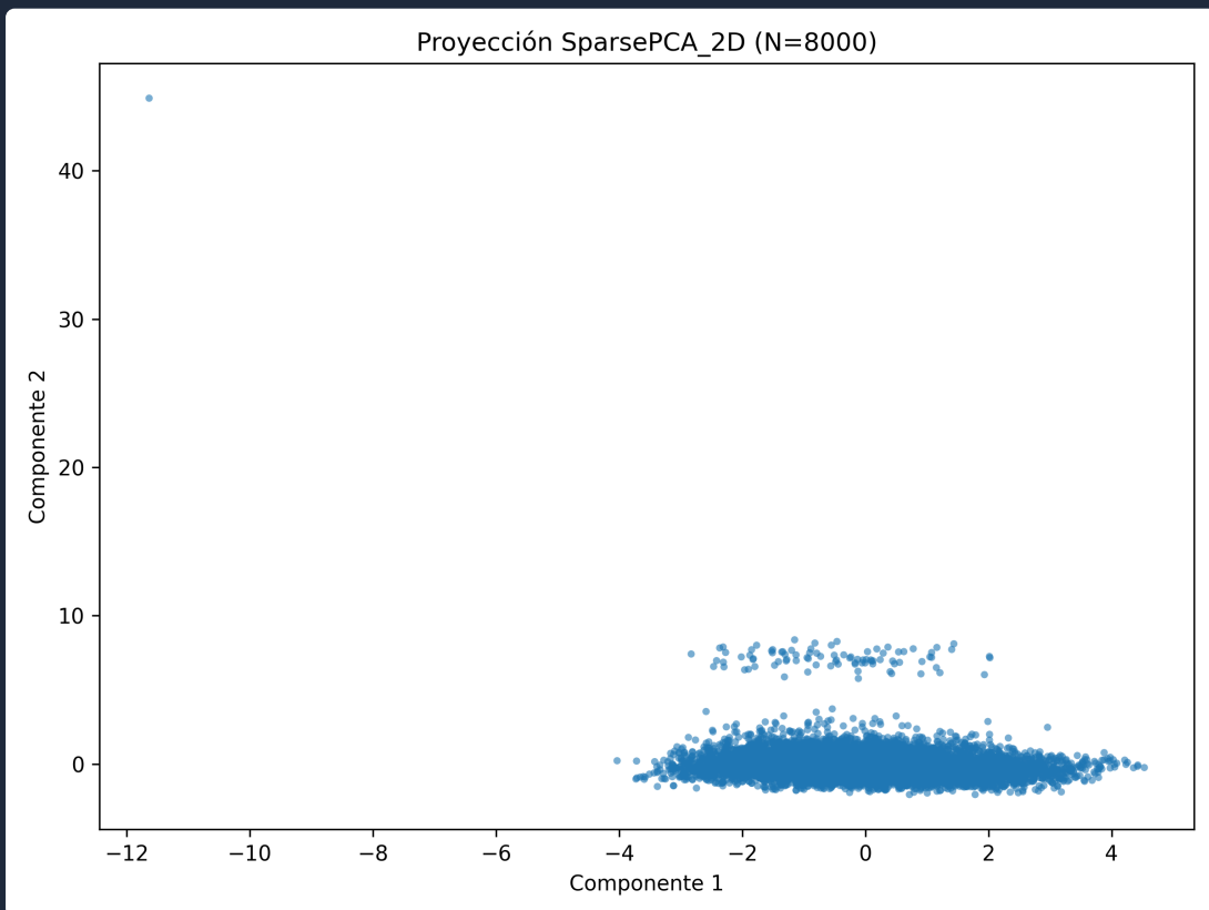
plot_SparsePCA_2D.png
