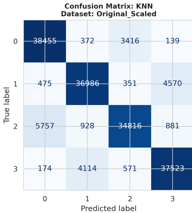
ConfusionMatrix_KNN_Original_Scaled.png
