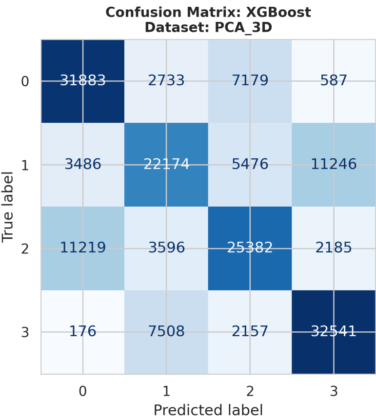
ConfusionMatrix_XGBoost_PCA_3D.png
