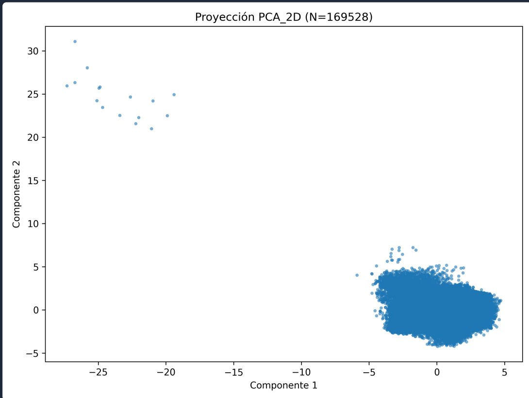
plot_PCA_2D.png
