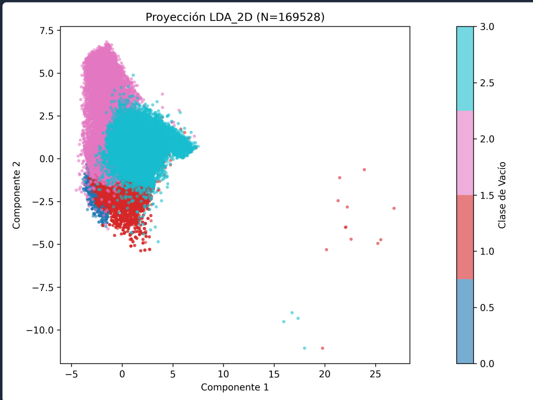
plot_LDA_2D.png
