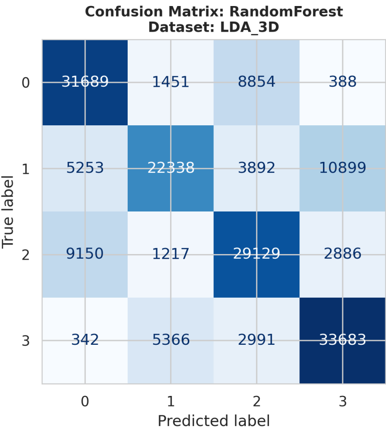
ConfusionMatrix_RandomForest_LDA_3D.png
