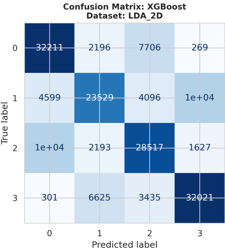
ConfusionMatrix_XGBoost_LDA_2D.png
