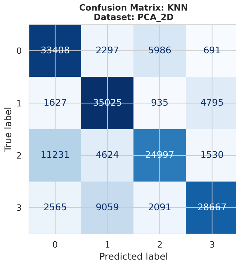
ConfusionMatrix_KNN_PCA_2D.png
