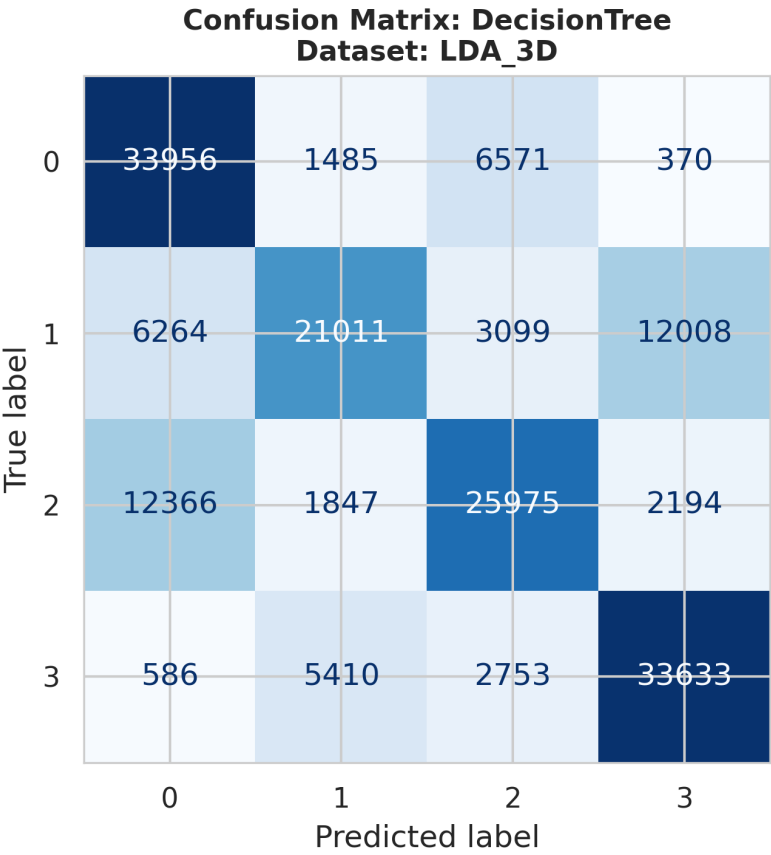
ConfusionMatrix_DecisionTree_LDA_3D.png
