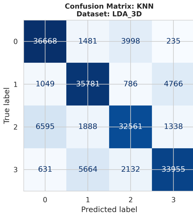
ConfusionMatrix_KNN_LDA_3D.png
