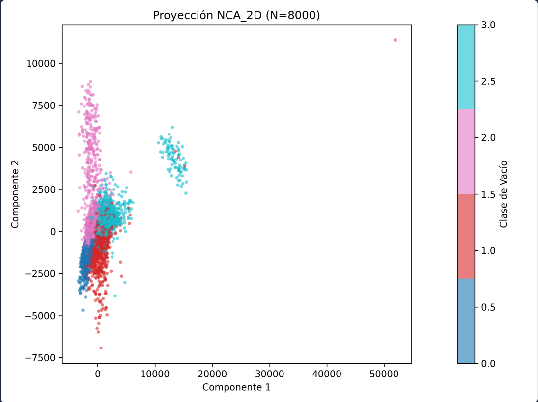
plot_NCA_2D.png
