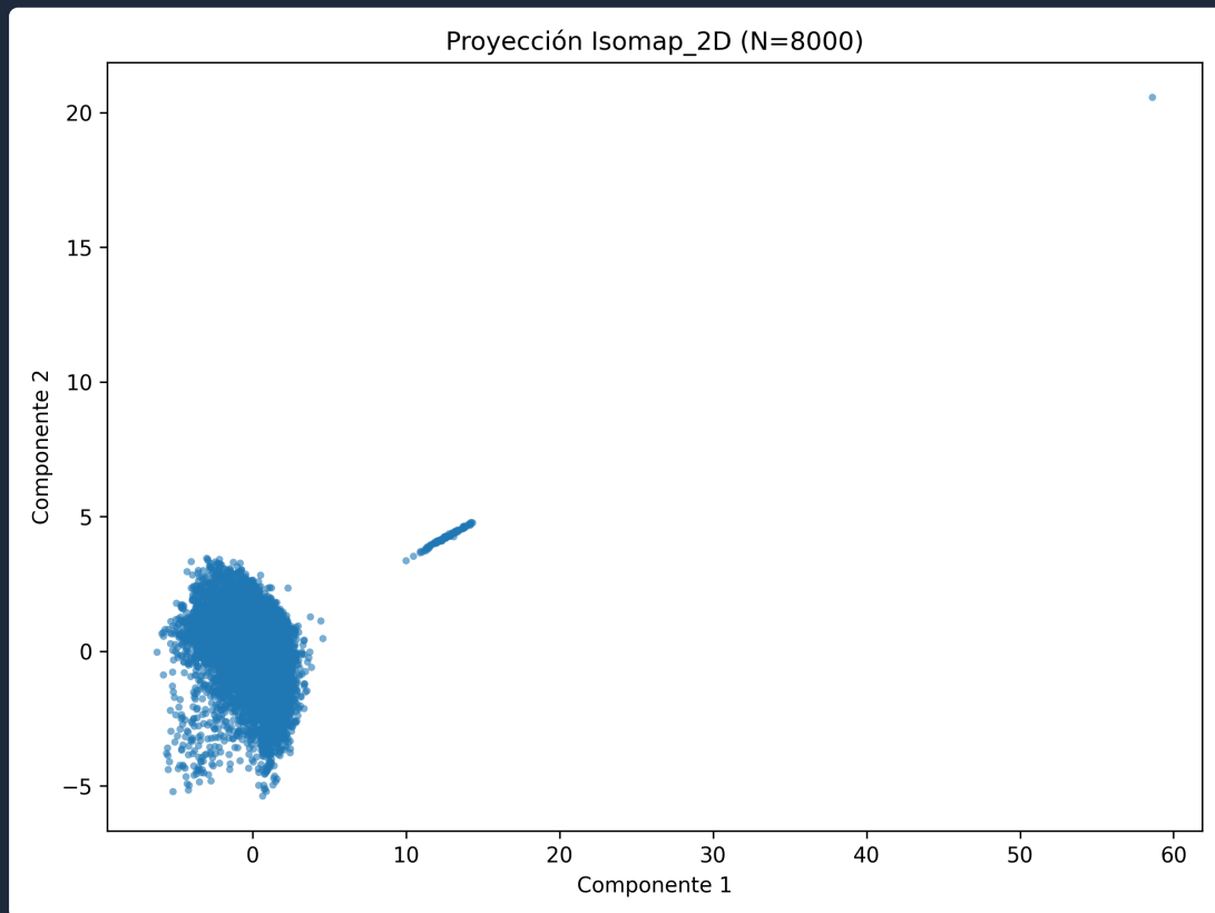
plot_Isomap_2D.png
