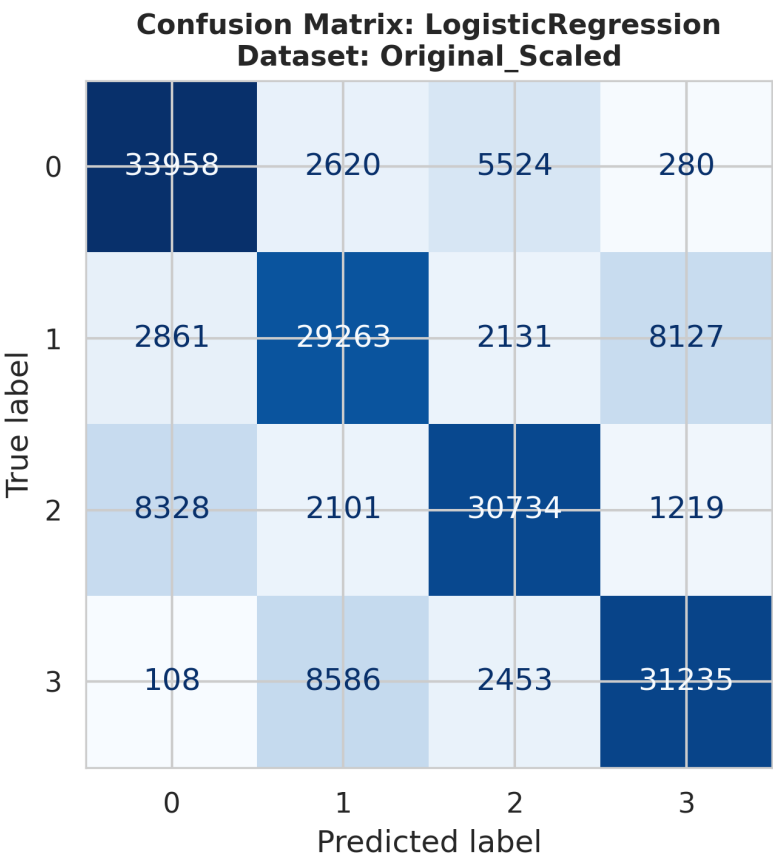
ConfusionMatrix_LogisticRegression_Original_Scaled.png
