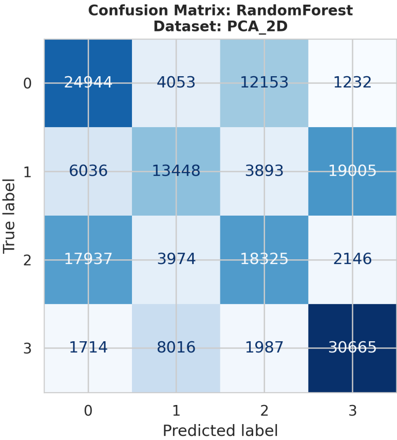
ConfusionMatrix_RandomForest_PCA_2D.png
